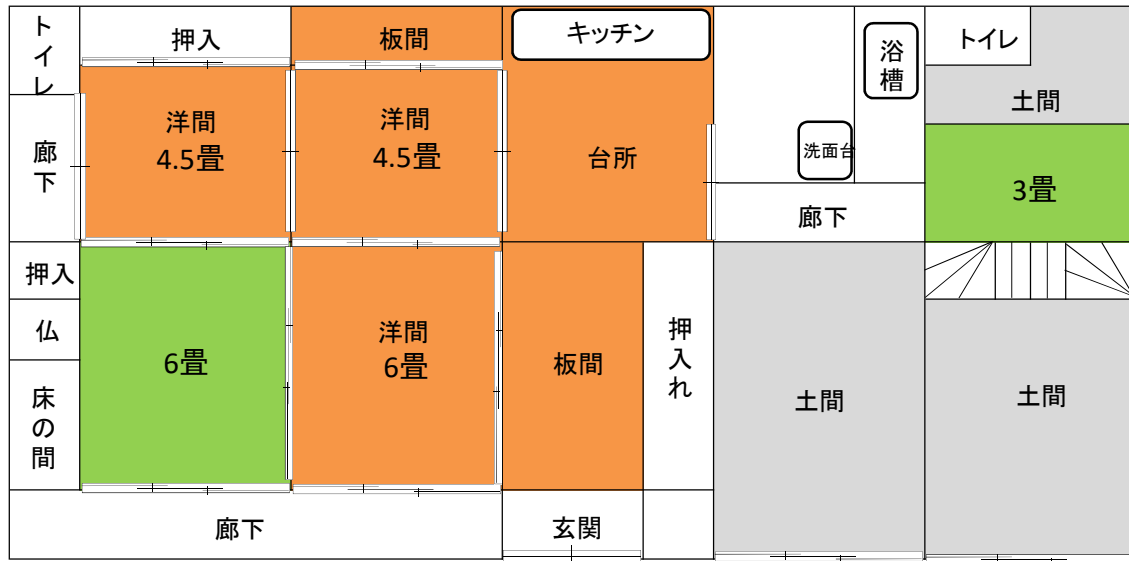
1階
